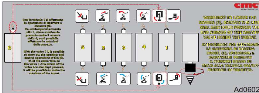
Afbeelding 78: noodmanoeuvres.
